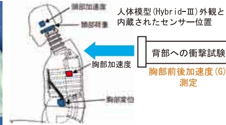
インパクタ衝突面・丸型 インパクタ質量 23.3 kg
